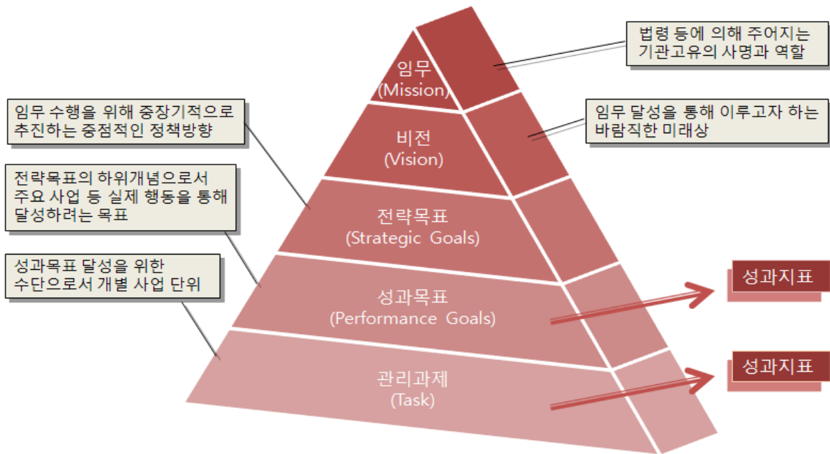
<성과관리 구성요소>
