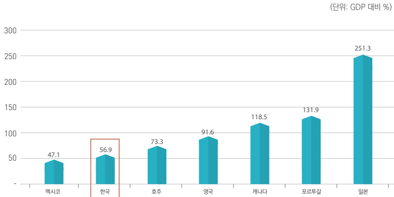
그림 5-14 D3의 국제비교
